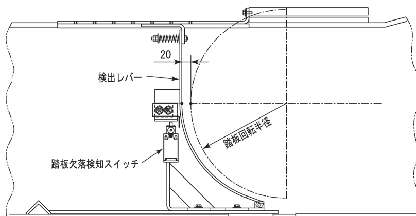
従動側
