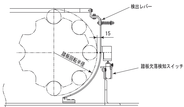
駆動機側
