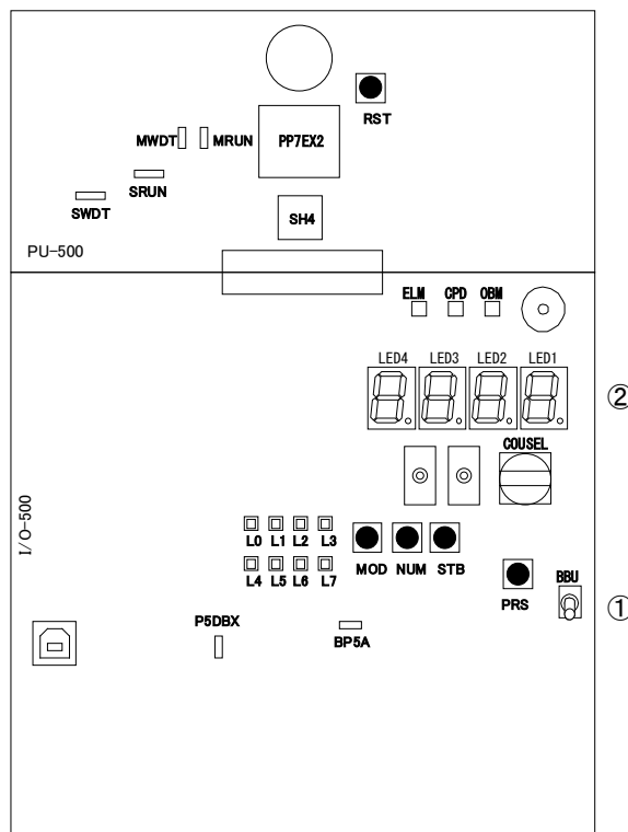
I/O 基板
