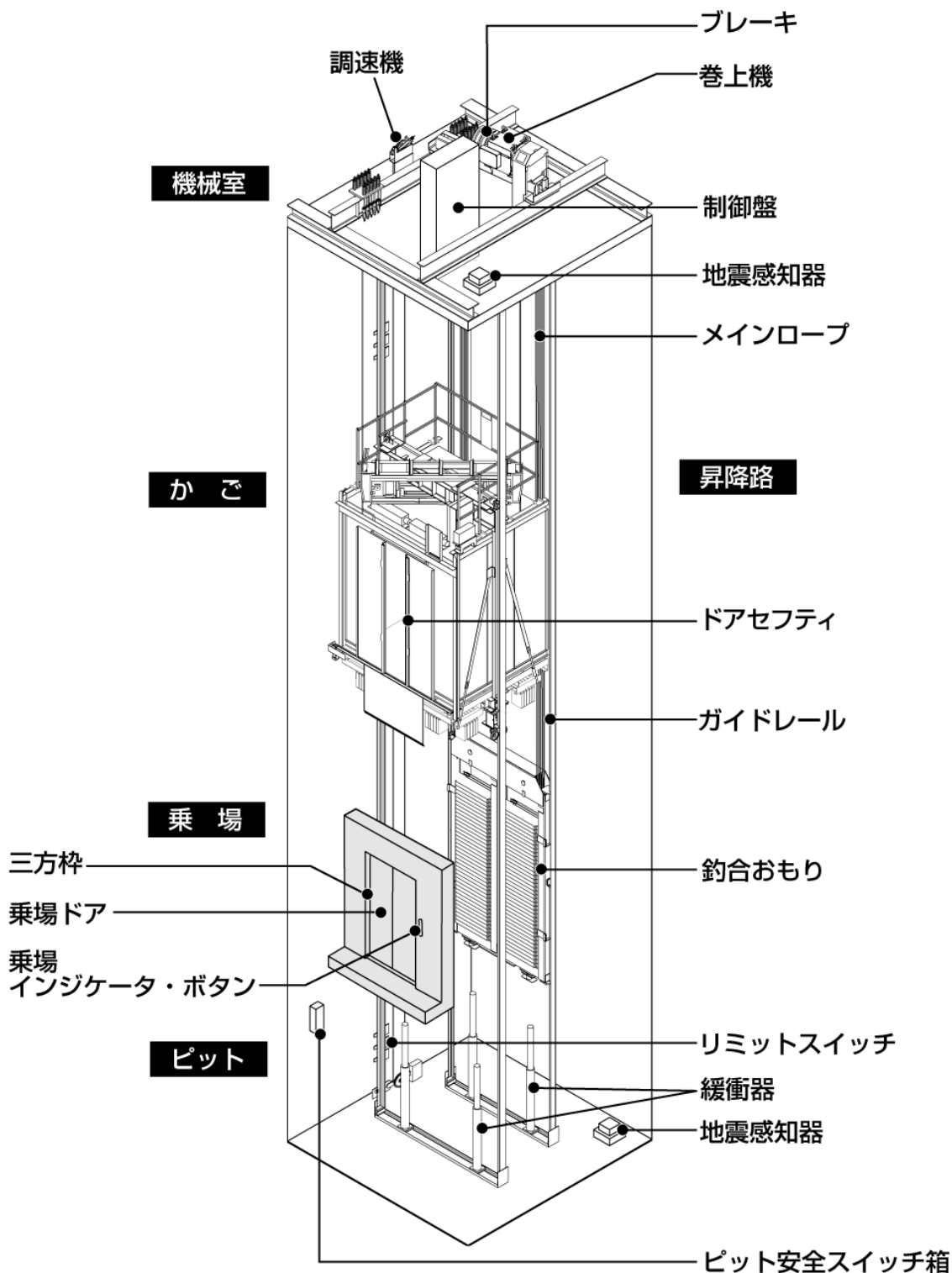
中低速エレベーターの場合
