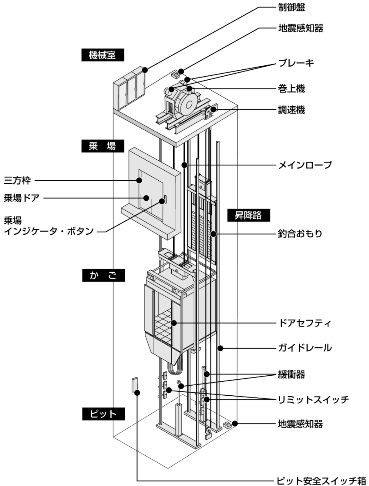
高速エレベーターの場合
