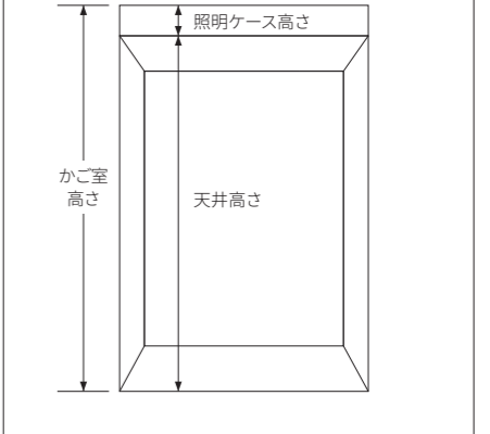
■天井高さとかご室高さの関係
