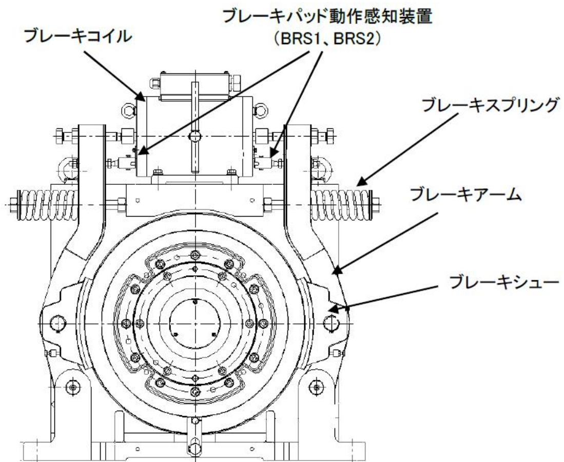
ブレーキ概略図
