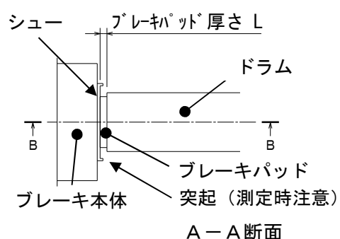
MX06 シリーズ、MX10 シリーズ、MX20 シリーズ ブレーキ概略図
