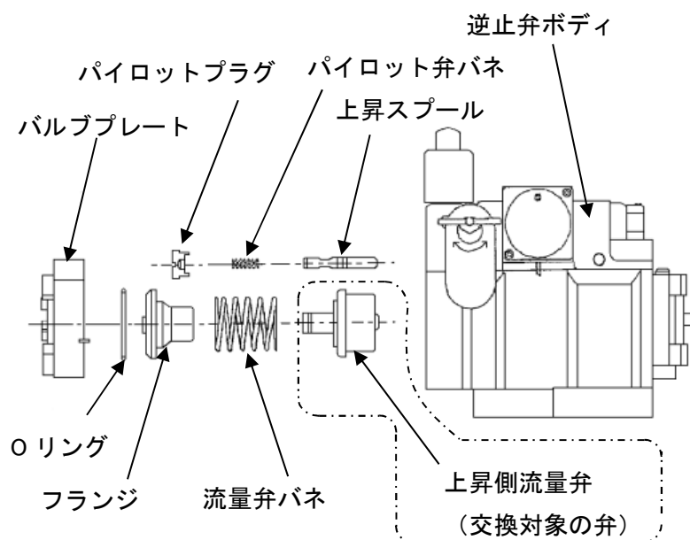
主たる逆止弁（上昇側流量弁）
