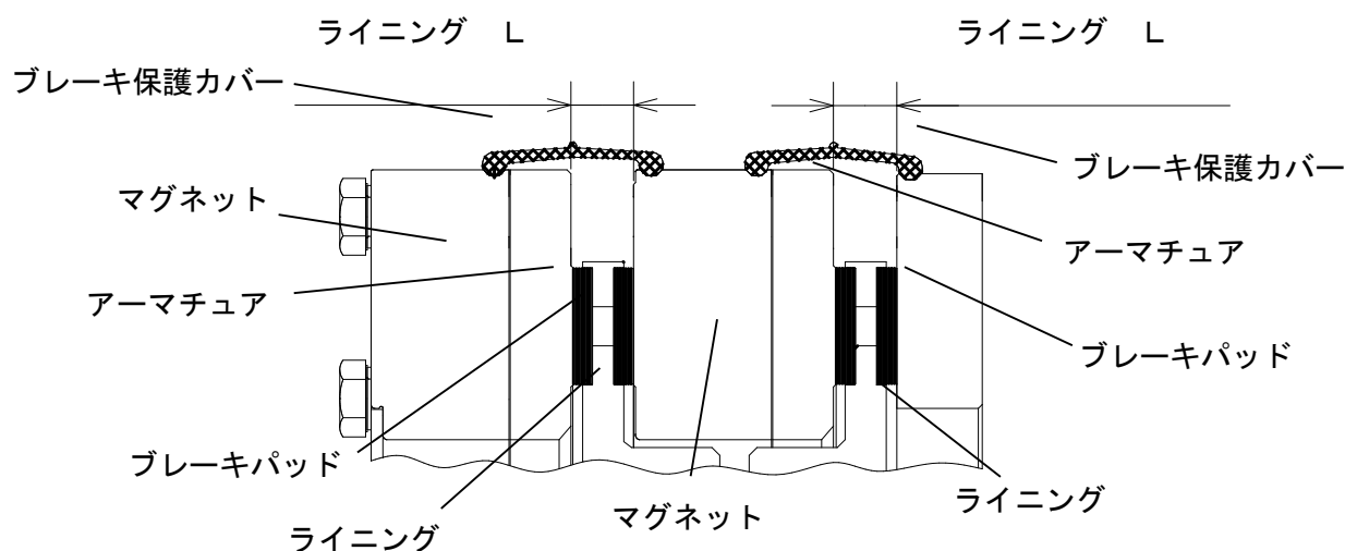
ブレーキ概略図（ダブルブレーキ）
