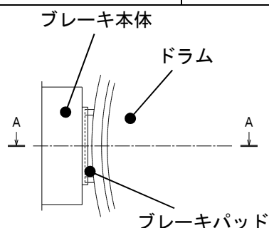
MX06 シリーズ、MX10 シリーズ、MX20 シリーズ ブレーキ概略図
