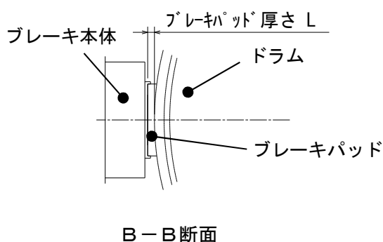
MX06 シリーズ、MX10 シリーズ、MX20 シリーズ ブレーキ概略図
