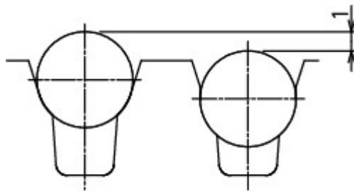
図3. 綱車溝間の摩耗差
