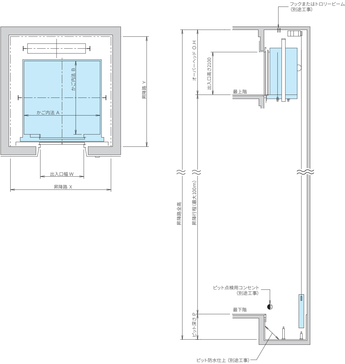
据付図
