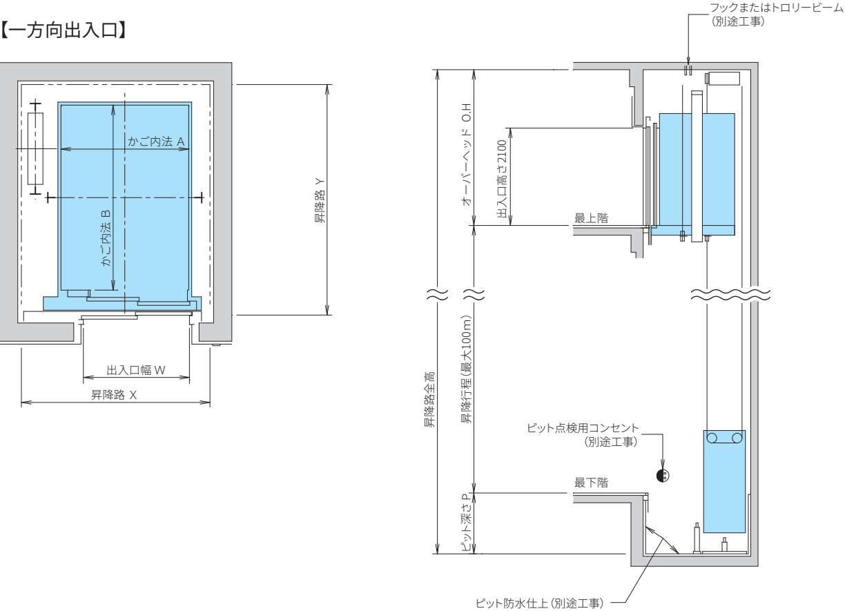
据付図
