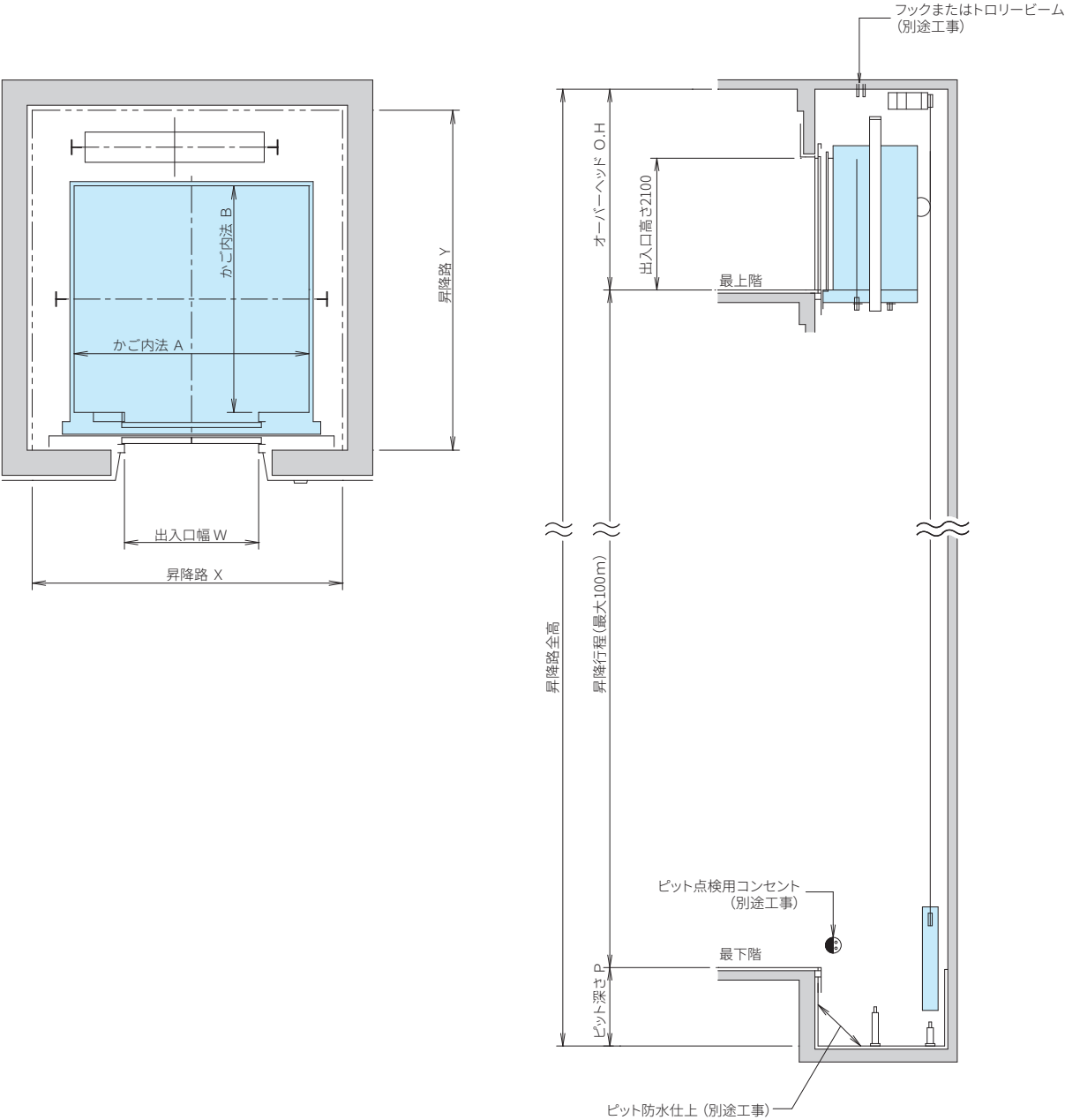
据付図
