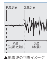
▲地震波の到着イメージ
