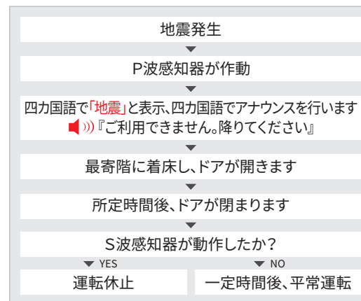
地震時最寄階停止
