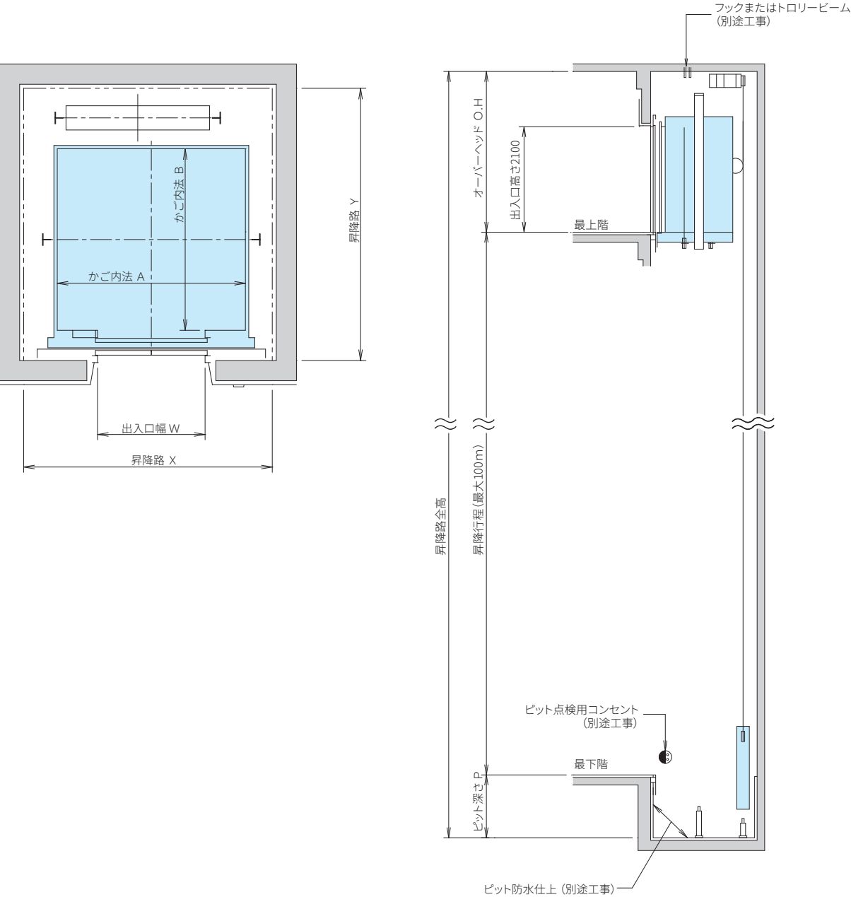
据付図
