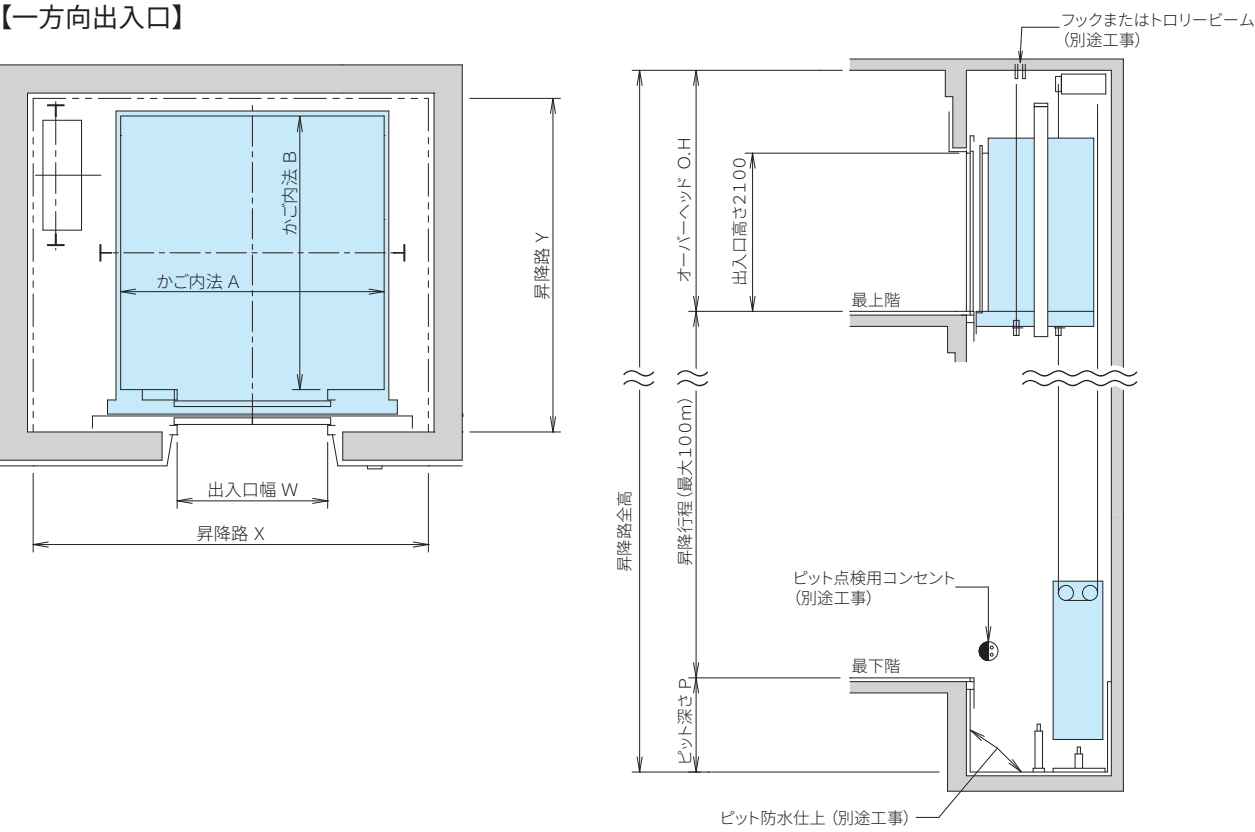
据付図
