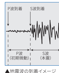
▲地震波の到着イメージ
