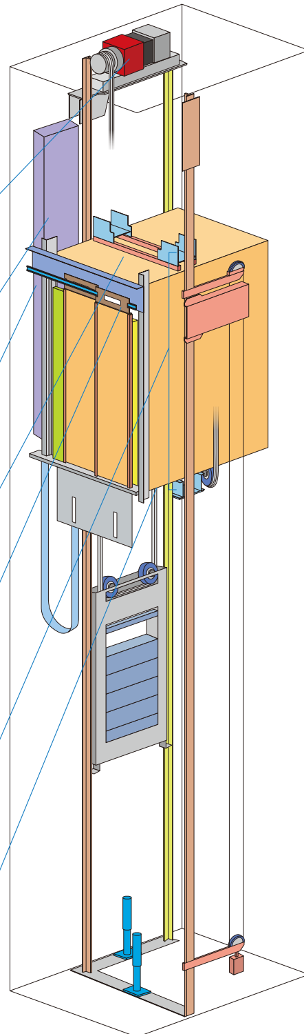
スぺーセルGR II住宅用R形 エレベーター構造図(イメージ図)
