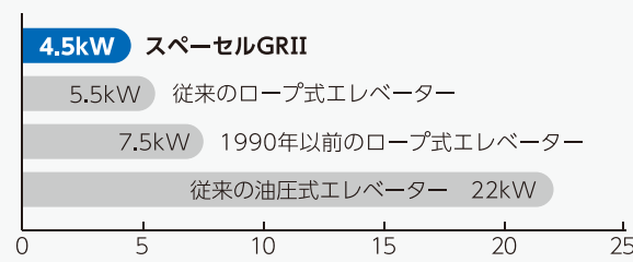
▲電動機容量の変遷(弊社比) 乗用11人乗り速度60m/minの場合
