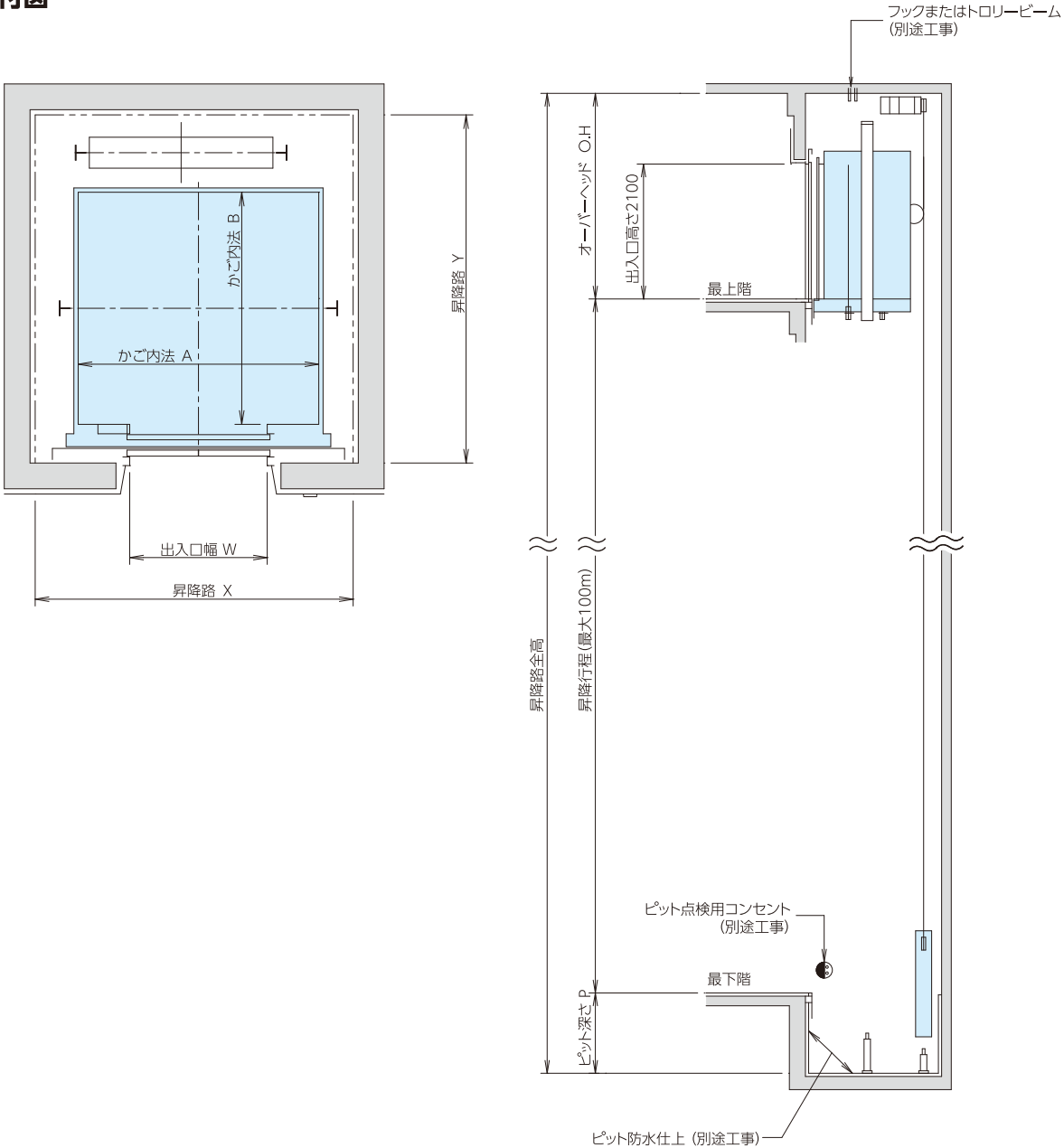
据付図
