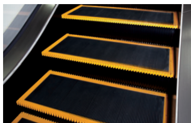
ご利用の方の安全に配慮し、階段の先端部分に緩衝材を採用した新しいエスカレーター階段
